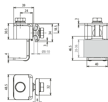
Maßbild AKK DUL 8.10 KBF 20 36 V2A
