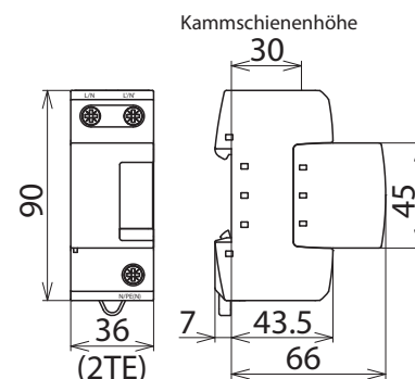
Maßbild DB M 1 150
