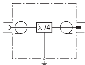
Prinzipialschaltbild DGA L4 7 16 MFA
