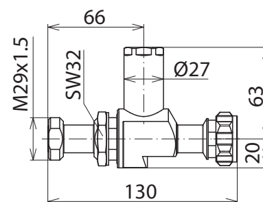
Maßbild DGA L4 7 16 MFA
