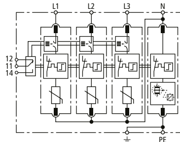
Prinzipialschaltbild DG M TT ACI 385 FM
