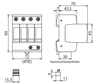
Maßbild DG M TT ACI 385 FM
