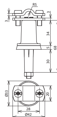
Maßbild DLH ZS 7.10 FL20 KT12 STTZN
