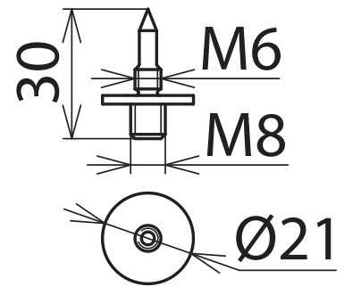
Maßbild EL M8 S PHE PHV
