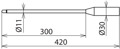
Maßbild
