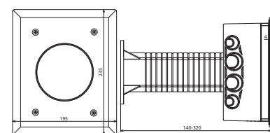
Maßbild
