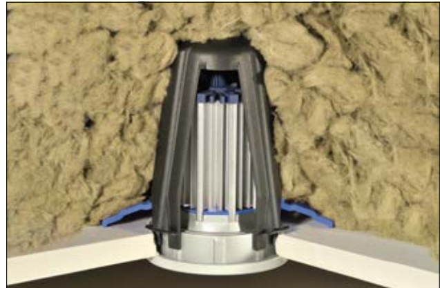
Die vier zusätzlichen Beine beim SpotClip-II ermöglichen den Einsatz von loser Hohlraumdämmung.
