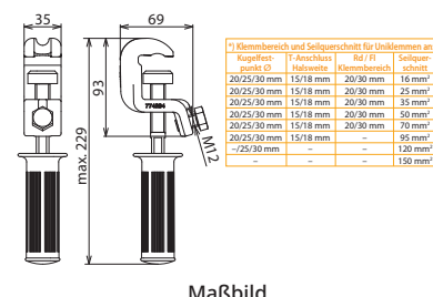
Maßbild
