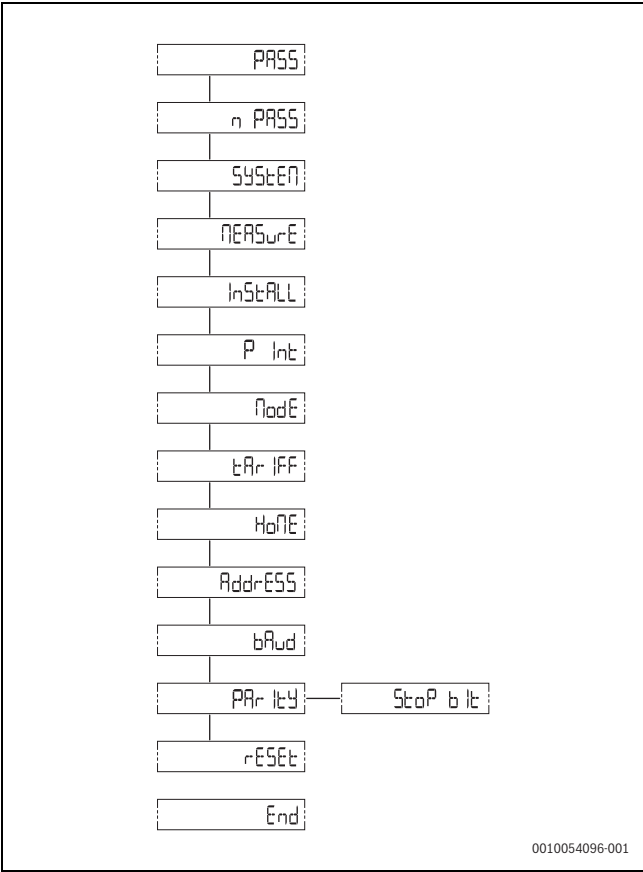
Fig. 189 Menu Paramètre de l'écran d'affichage
