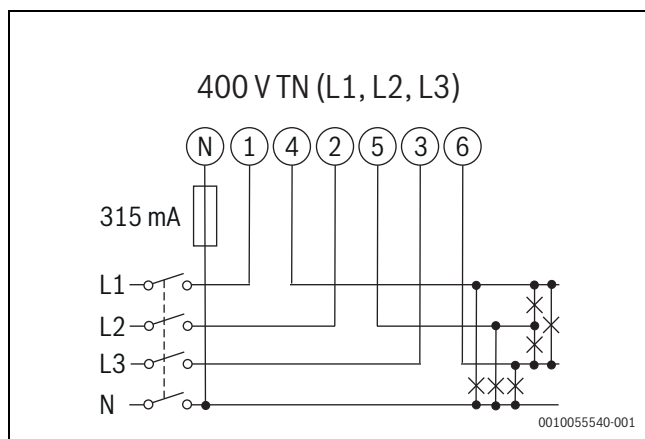
Sl.442 Shema trifaznega sistema, 4 žice (400 V TN)
