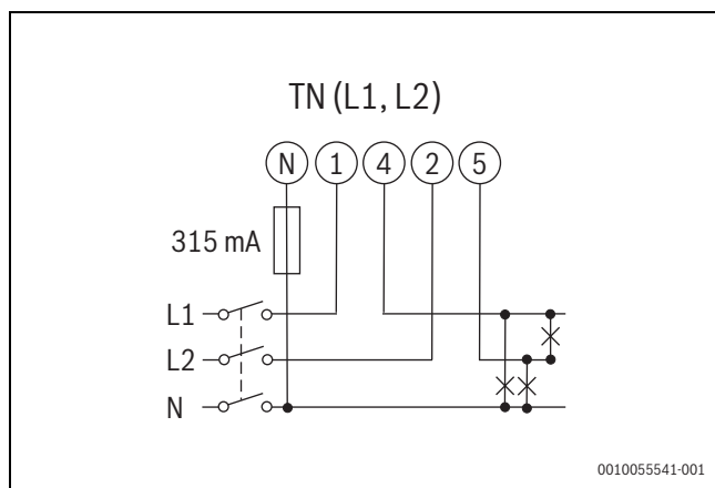
sl. 405 Trofazni sistem Dijagram, 3-žičani(TN)
