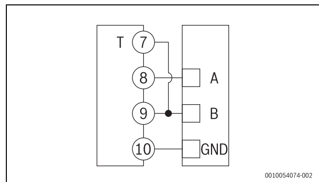
sl. 408 Dijagram RS485 Modbus sa Master jedinicom
