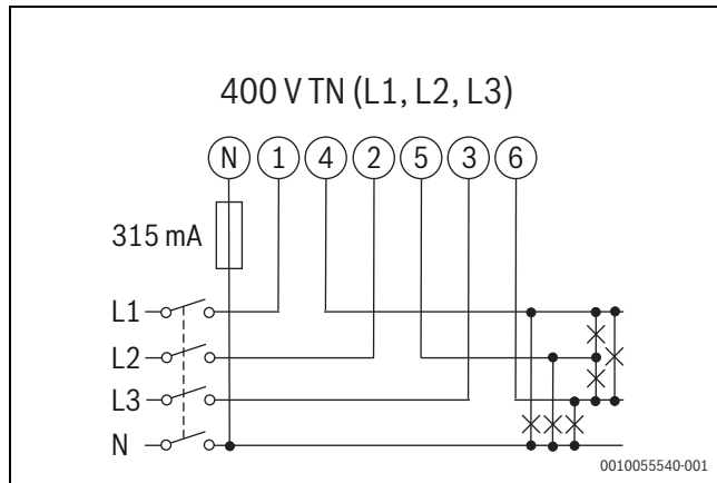
Bild 62 Anschlussplan Dreiphasensystem, 4 Leiter (400 V TN)
