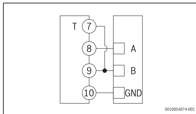
Фиг. 9 Схема на RS485 Modbus c Master
