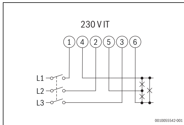
Obr. 26 Graf třífázového systému, třívodičového (230 V IT)
