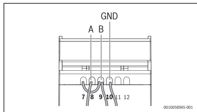
sl. 409 GND veza
