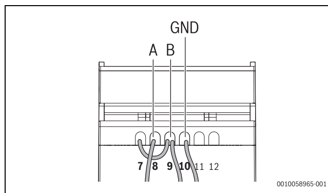
Fig. 371 Conexão GND
