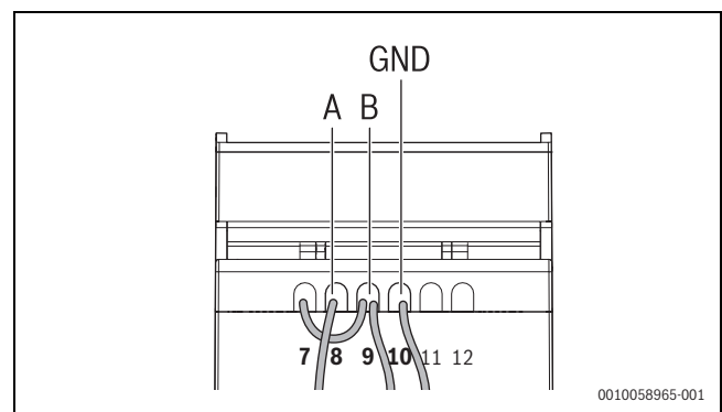
Fig. 238 Connessione GND
