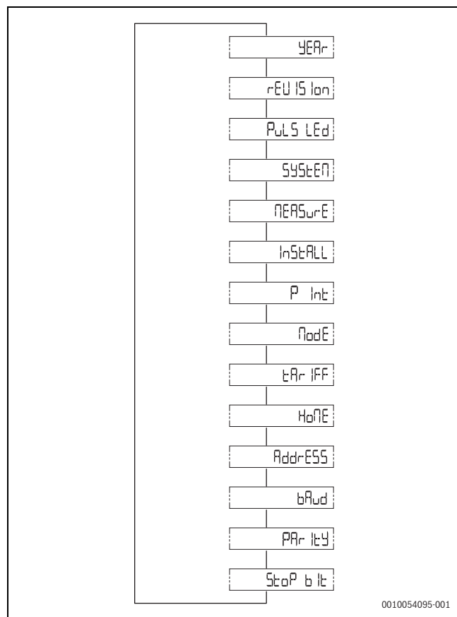
sl. 418 Meni sa informacijama ekrana sa prikazom
