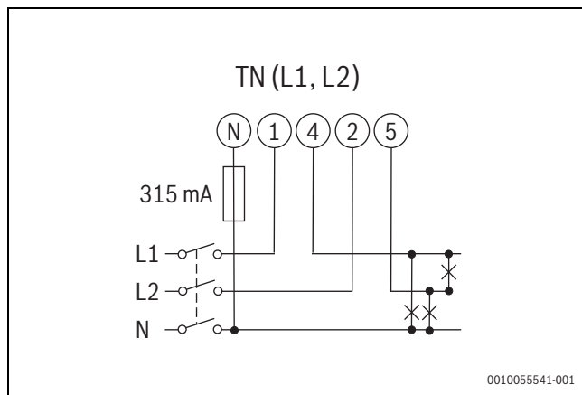
Bild 63 Anschlussplan Zweiphasensystem, 3 Leiter (TN)
