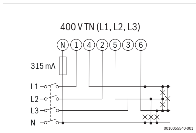
Fig. 366 Diagrama do sistema trifásico, 4 condutores (400 V TN)
