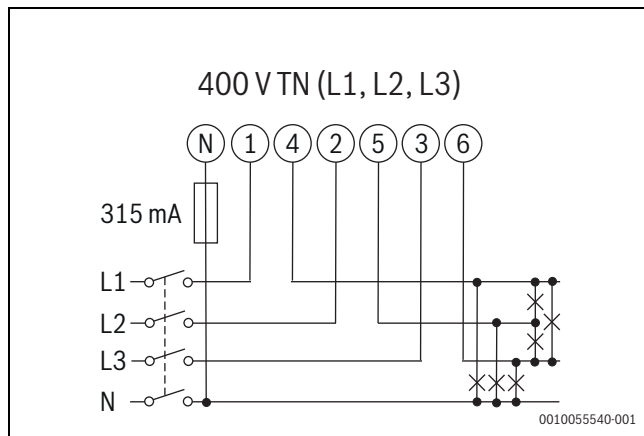
Fig. 43 Diagram over trefaset system, 4-ledninger (400 V TN)
