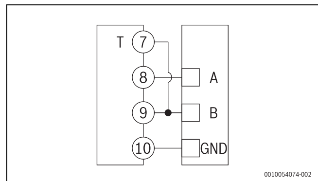
Bild 66 Anschlussplan RS485 Modbus mit Master
