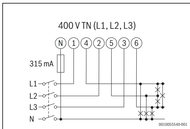
Σχ. 81 Διάγραμμα τριφασικού συστήματος, 4 καλώδια (400 V TN)
