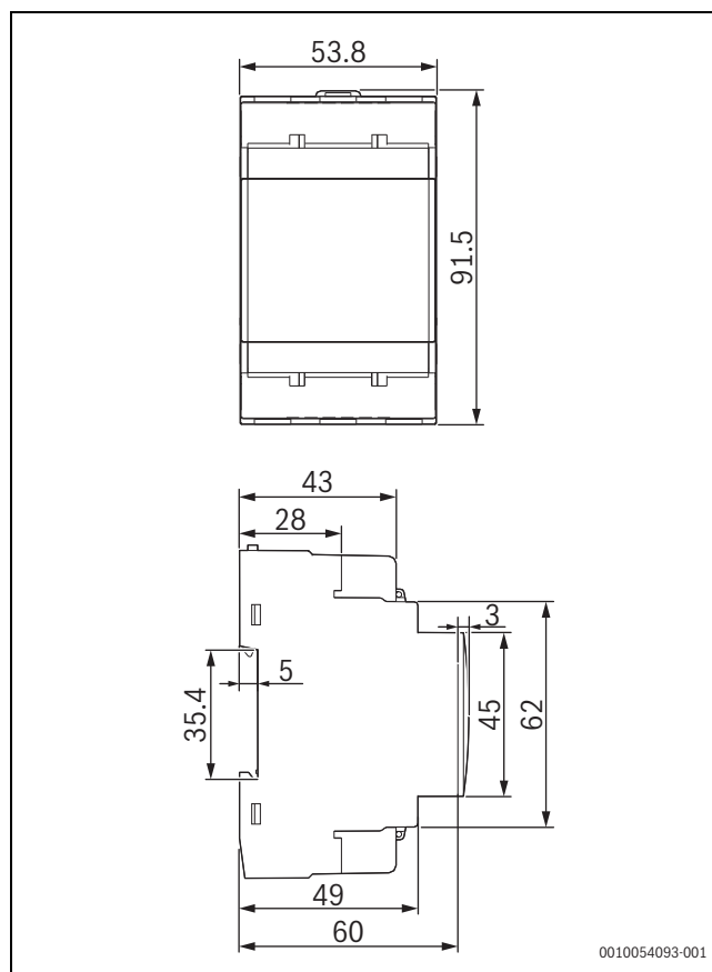
Joon. 137 Toote mõõtmed
