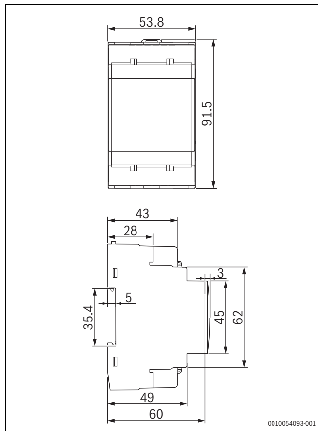
Мал. 479 Розміри виробу
