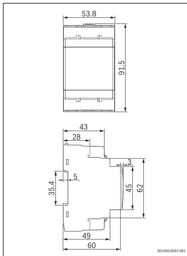
Att. 251 Izstrādājuma izmēri
