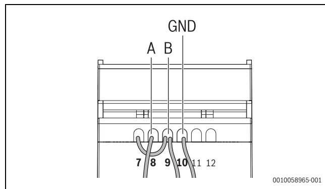
Afb. 295 GND-verbinding
