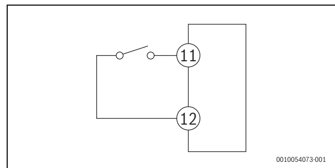
Fig. 46 Diagram for digital indgang
