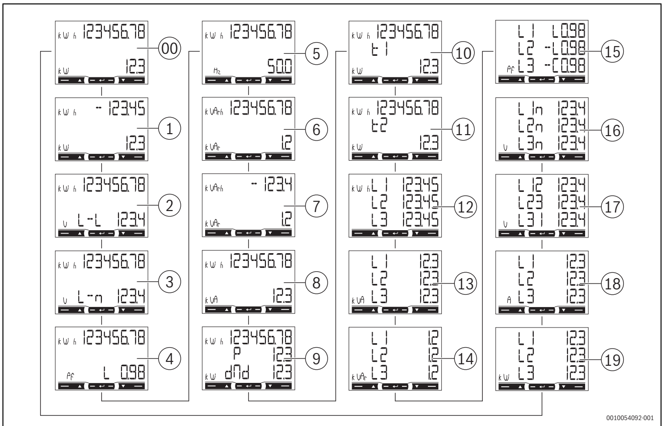
Afb. 321 Meetwaardepagina's van het display
