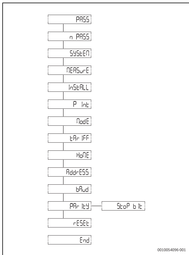
Rys. 360 Menu parametrów ekranu wyświetlacza
