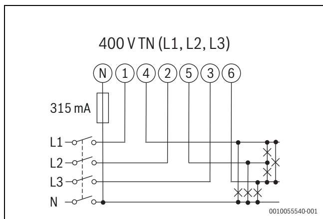
Afb. 309 Driefase systeem diagram, 4-draads (400 V TN)
