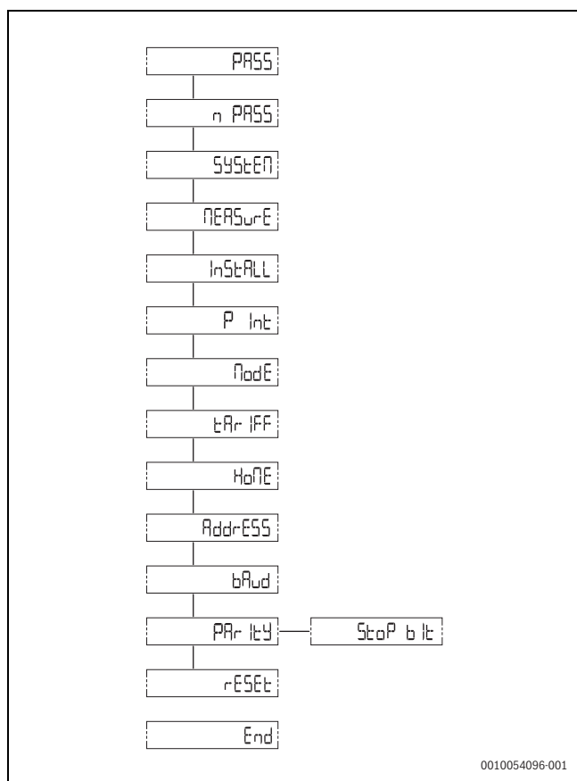
Bild 75 Parametermenü des Displays
