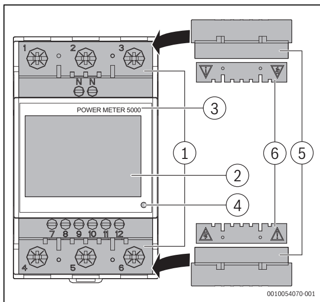
Obr. 420 Prehľad výrobku
