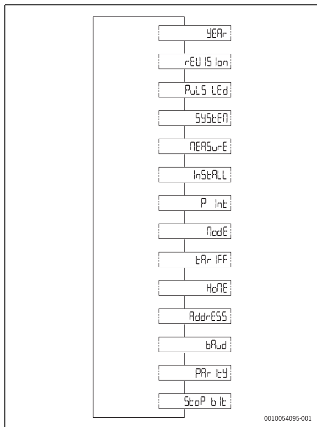
Pav. 285 Ekrano informacijos meniu
