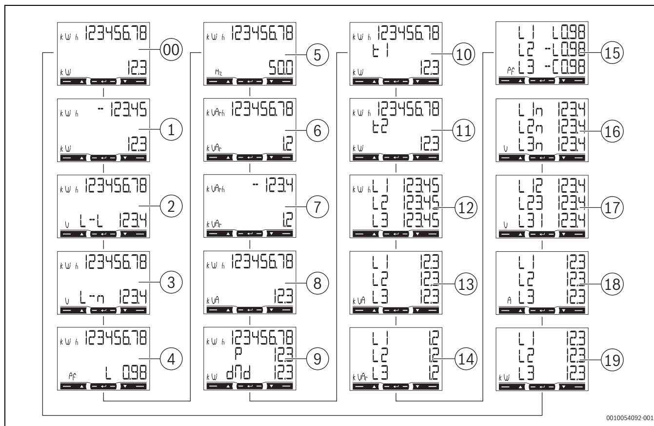
Fig. 397 Pagini de măsurare ale ecranului de afisare
