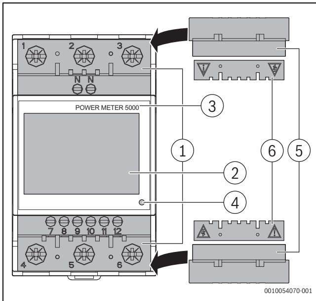
Bild 59 Produktübersicht
