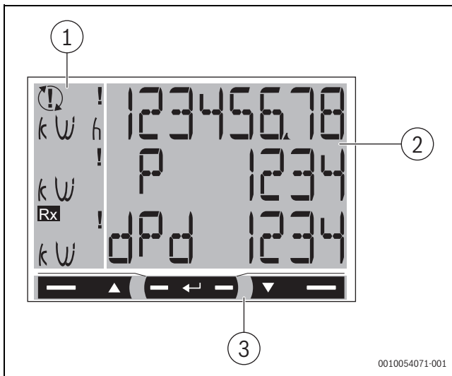
Bild 60 Produktübersicht
