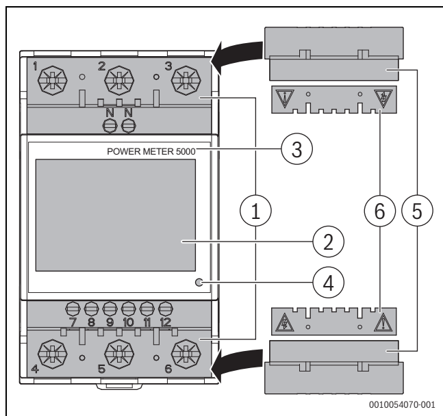
Sl.439 Pregled sestavnih delov izdelka
