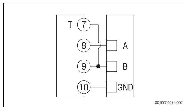
Fig. 332 RS485 Modbus-masterdiagram
