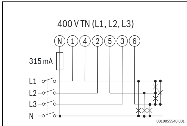
Kuva 157 Kolmivaiheinen järjestelmäkaavio, 4 johdinta (400 V TN)
