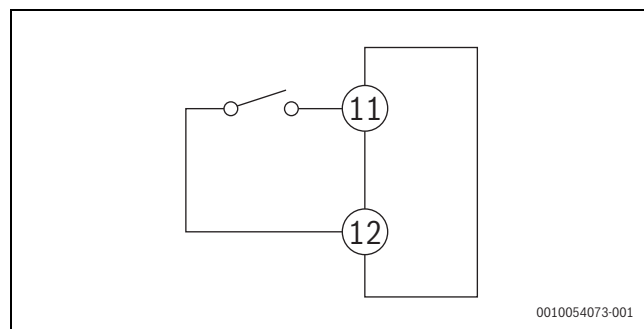
Afb. 293 Digitale input schema
