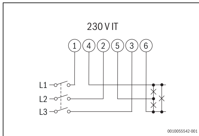
216. ábra Háromfázisú rendszer diagram, 3 vezetékes (230 V IT)
