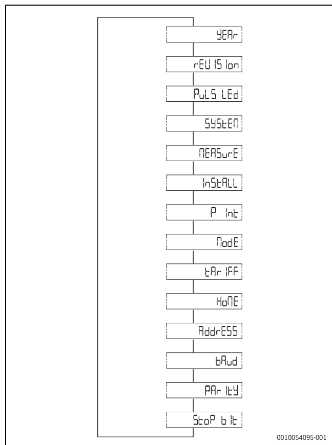
Sl.209 Informacijski izbornik na zaslonu
