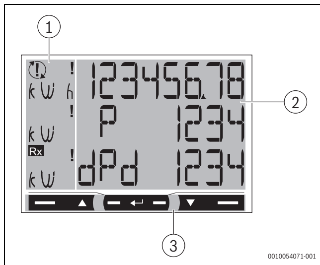
Afb. 288 Productoverzicht
