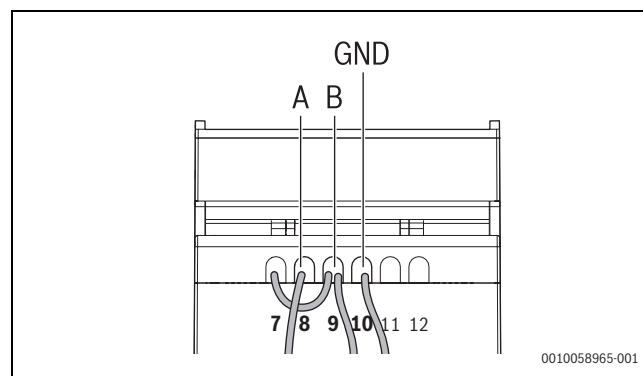
Rys. 352 Połączenie GND
