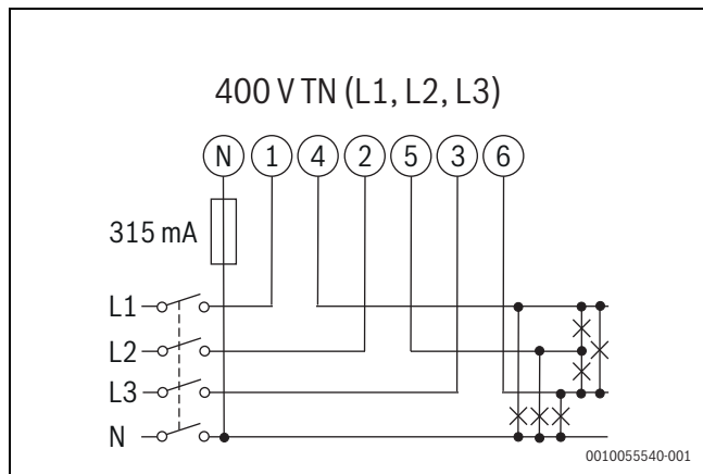
Pav. 271 Trifazės sistemos diagrama, 4 laidai (400 V TN)
