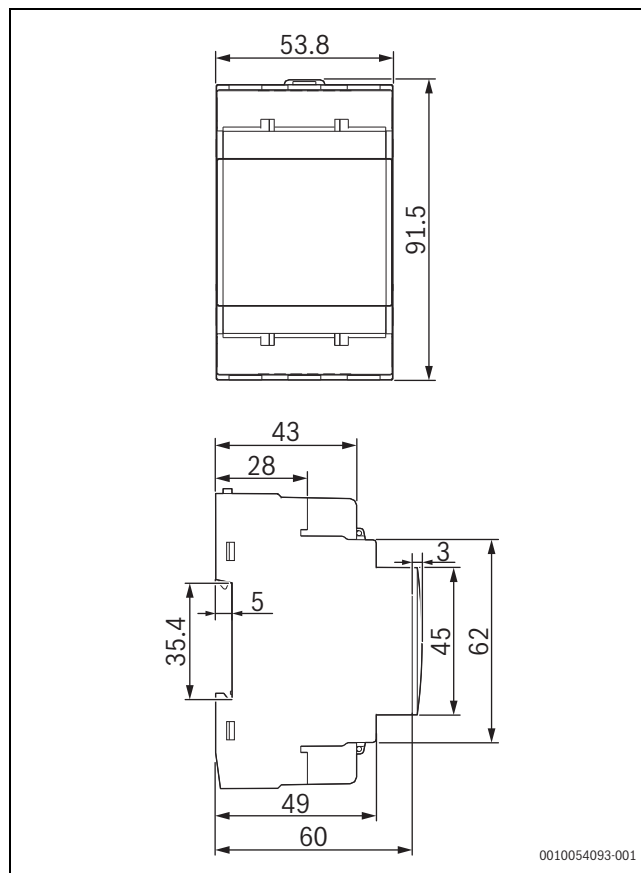
Sl.441 Dimenzije izdelka
