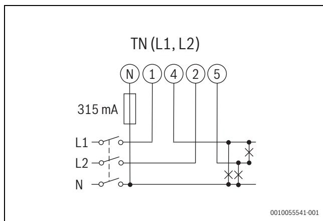
Fig. 44 Diagram over tofaset system, 3-ledninger (TN)
