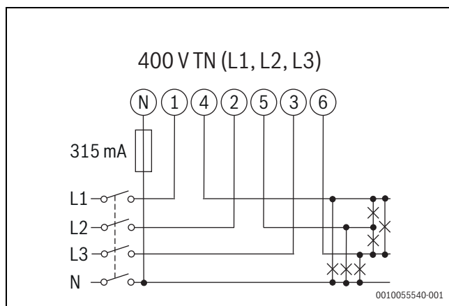
Fig. 119 Diagrama del sistema trifásico, 4 conductores (400 V TN)
