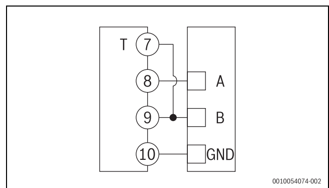
Fig. 237 Schema master RS485 Modbus
