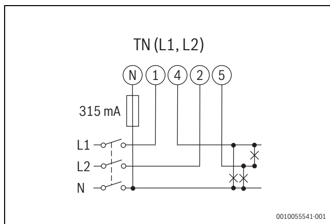
Fig. 234 Schema dell'impianto bifase, 3 fili conduttori (TN)
