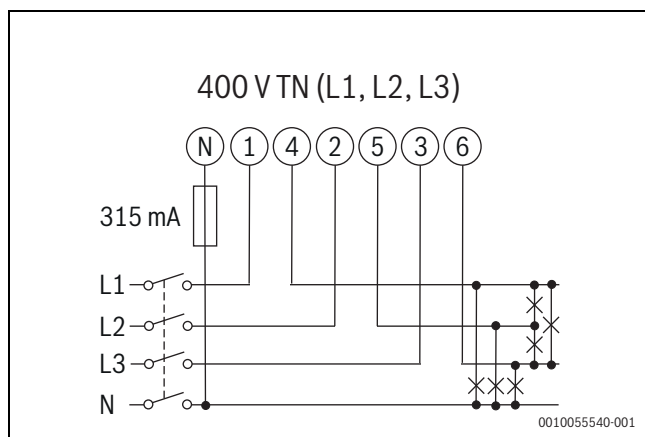
Fig. 385 Diagramă sistem trifazat, cu 4 fire (400 V, TN)
