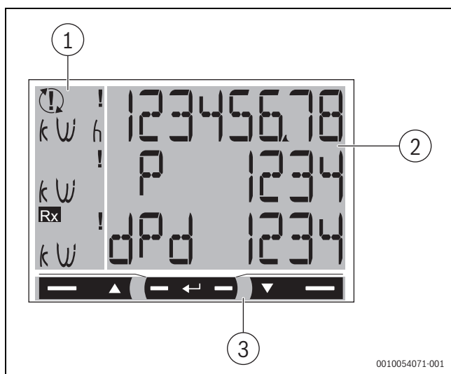
Fig. 231 Panoramica sul prodotto
