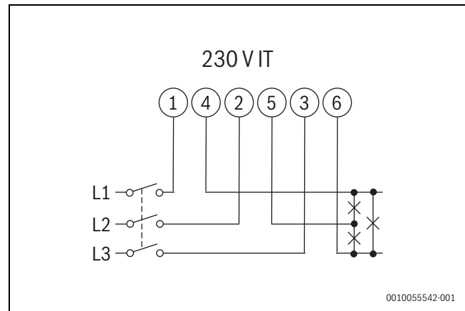
sl. 406 Trofazni sistem Dijagram, 3-žičani(230 V IT)
