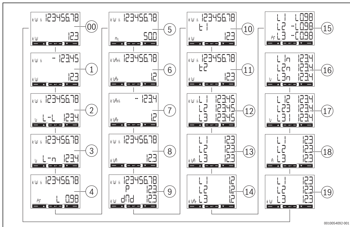
Fig. 245 Pagine dei valori di misura sullo schermo del display
