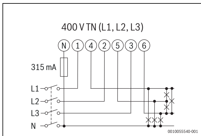
Fig. 328 Skjema for trefasesystem, 4 ledere (400 V TN)
