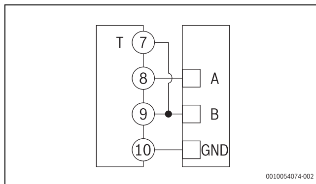
Att. 256 RS485 Modbus vedējsistēmas shēma
