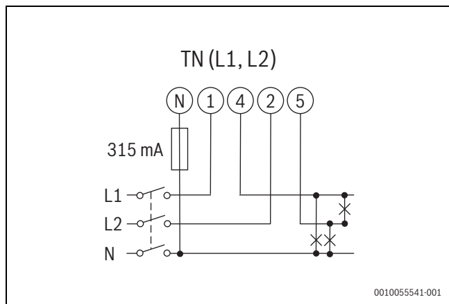
Pav. 272 Dvifazės sistemos diagrama, 3 laidai (TN)
