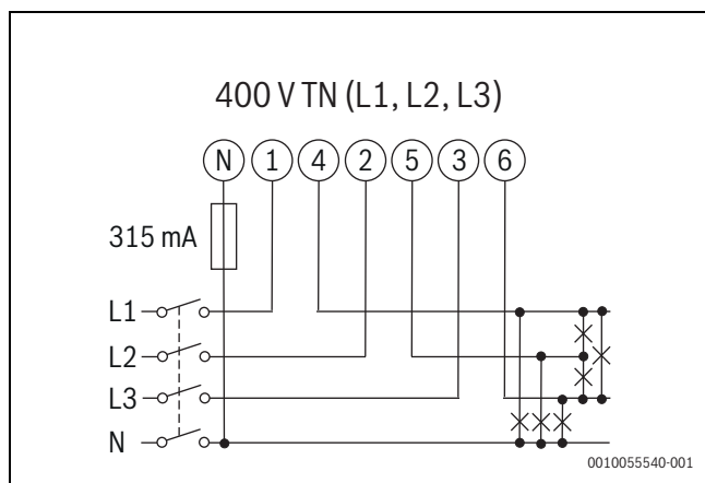
Afb. 290 Driefase systeem diagram, 4-draads (400 V TN)
