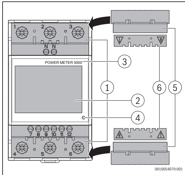
Afb. 287 Productoverzicht
