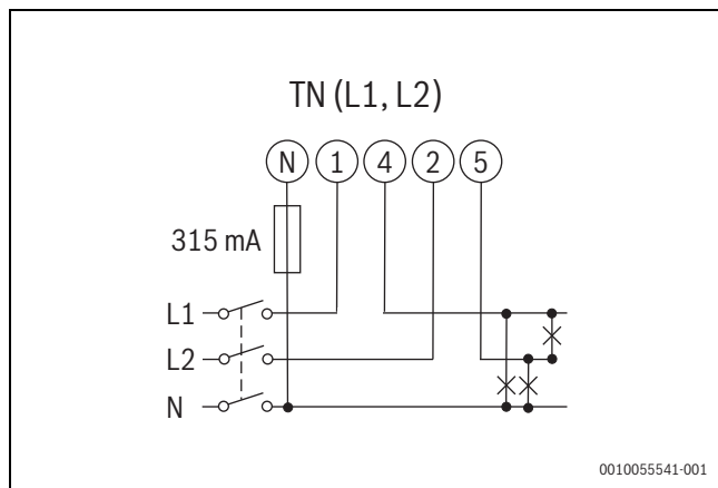
Obr. 25 Graf dvoufázového systému, třívodičového (TN)
