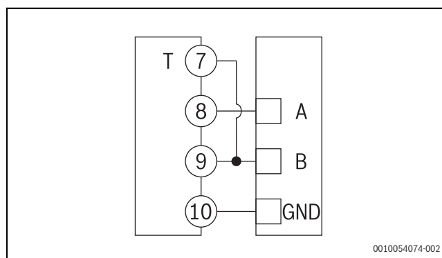
Fig. 370 Diagrama da unidade principal Modbus RS485
