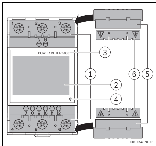
Obr. 21 Přehled výrobku
