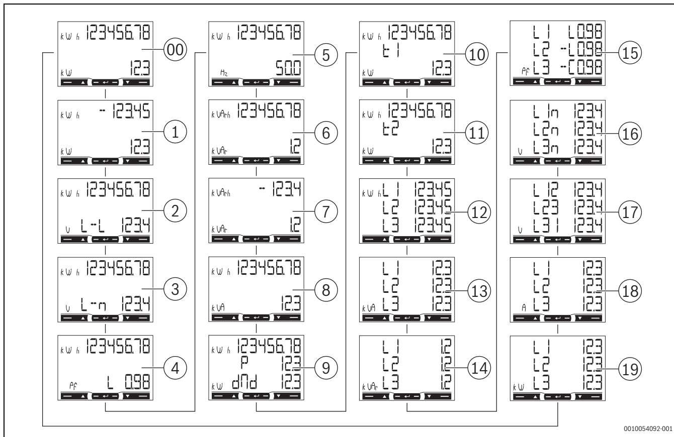
Fig. 378 Páginas de valor de medição do ecrã de visualização
