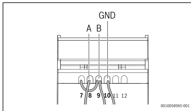
Sl.200 GND veza
