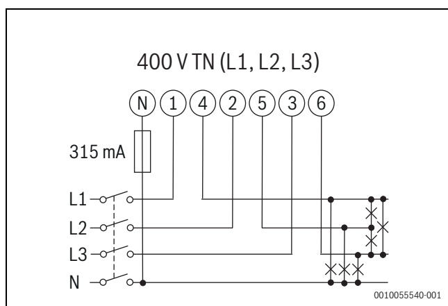
Rys. 347 Schemat systemu trójfazowego, 4-żyłowy (400 V TN)
