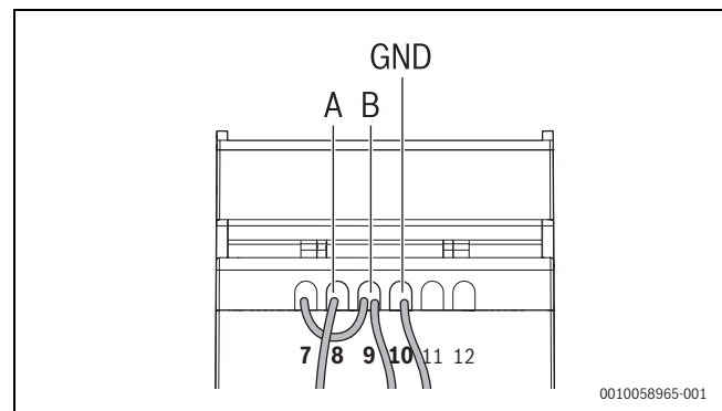
Kuva 162 Maadoitusliitäntä
