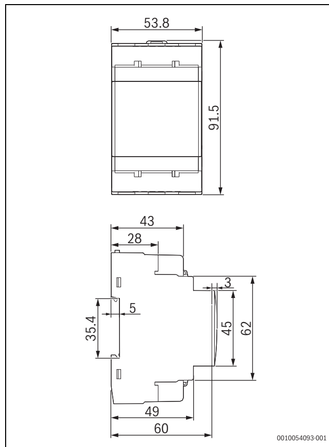
Fig. 42 Produktdimensioner
