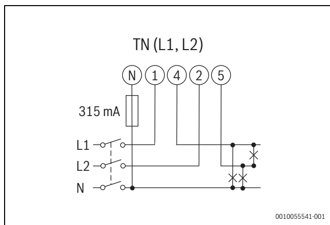
Sl.443 Shema dvofaznega sistema, 3 žice (TN)
