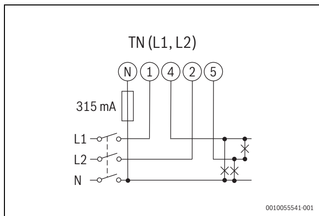
Sl.196 Shema dvofaznog sustava, 3-žilni (TN)
