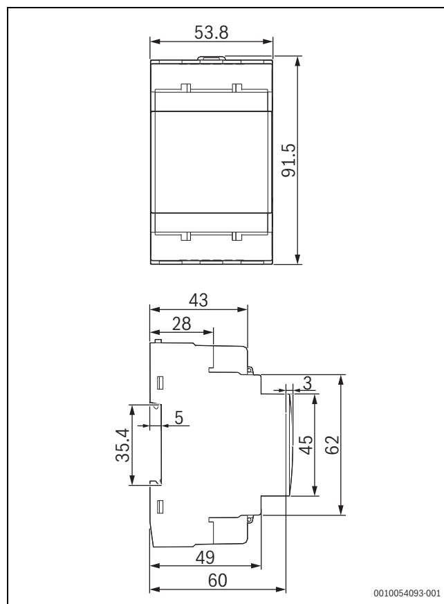
Sl.194 Dimenzije proizvoda
