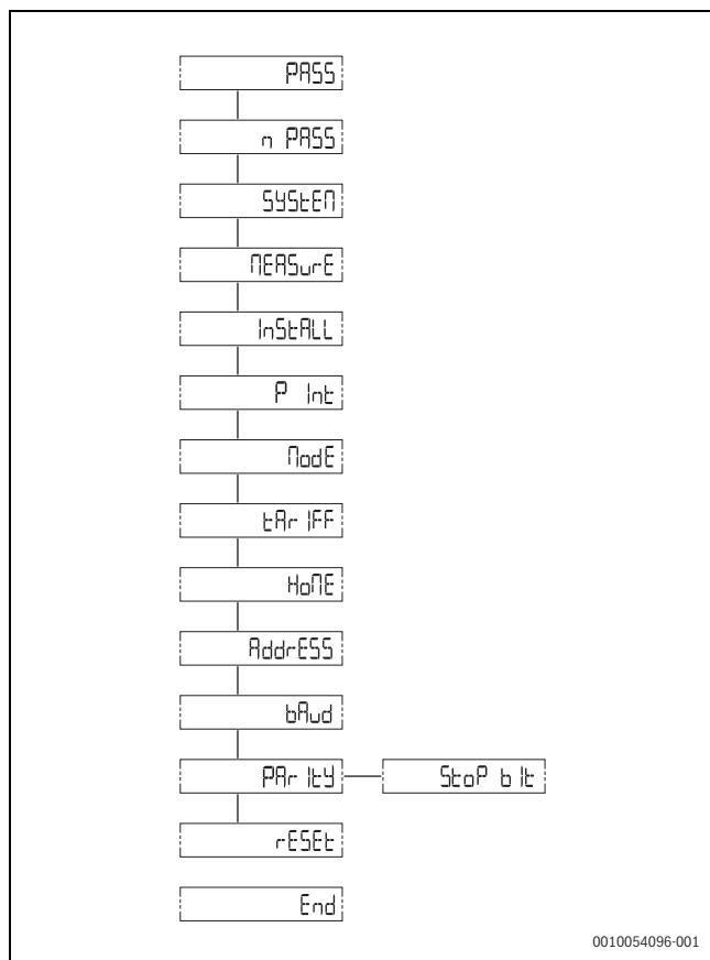
Obr. 436 Ponuka parametrov obrazovky displeja
