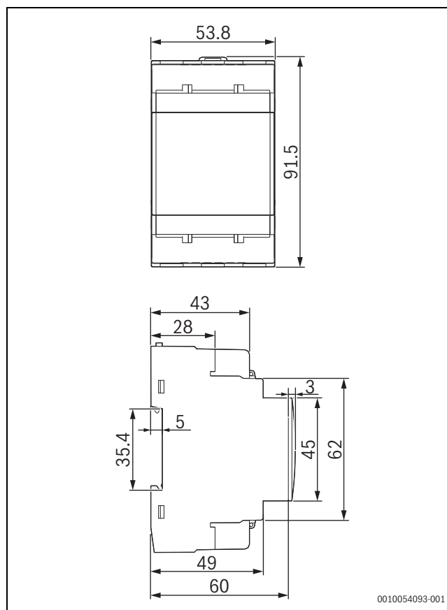
Fig. 327 Produktdimensjoner
