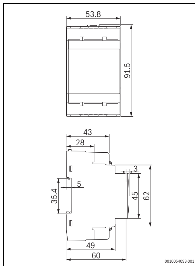
Fig. 175 Dimensions du produit
