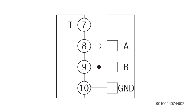
Fig. 180 Schéma Modbus RS485 maître
