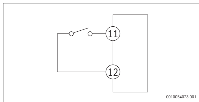
Att. 255 Digitālās ievades shēma
