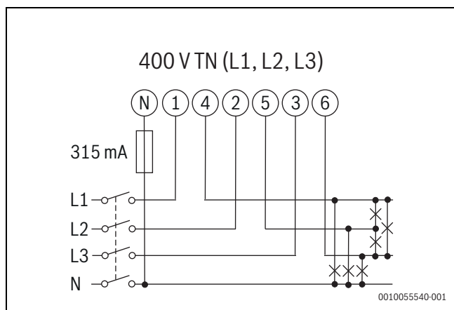
Мал. 480 Схема з'єднань трифазної системи, 4 жили (400 В TN)
