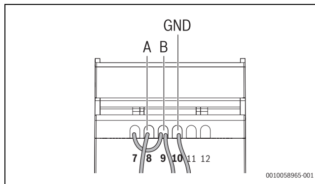
Afb. 314 GND-verbinding
