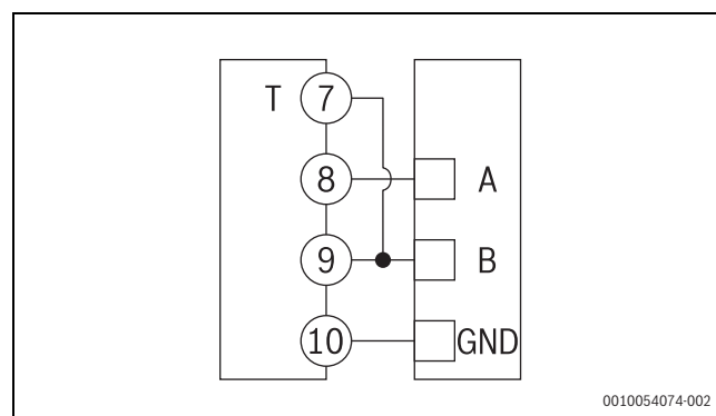
Rys. 351 Schemat Modbus RS485 z jednostką główną
