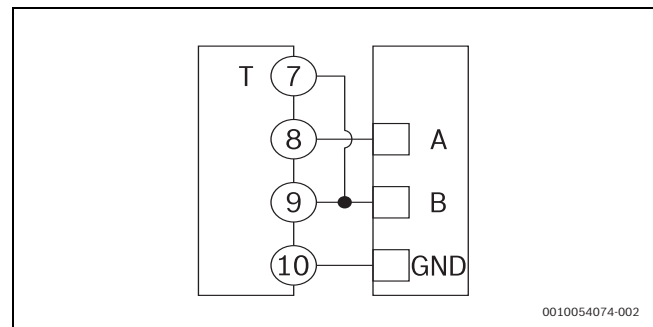
Kuva 161 RS485 Modbus Master -kaavio
