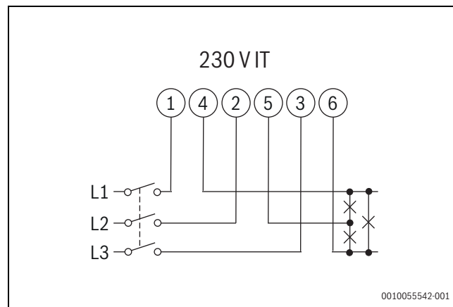
Fig. 330 Skjema for trefasesystem, 3 ledere (230 V IT)
