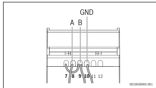
Bild 67 GND-Verbindung
