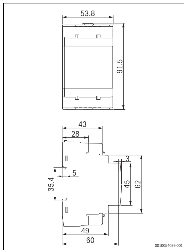
Obr. 422 Rozmery výrobku
