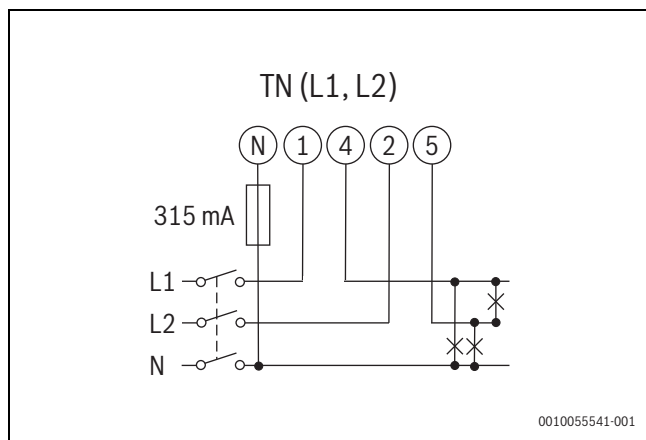
Afb. 291 Tweefase systeem diagram, 3-draads (TN)
