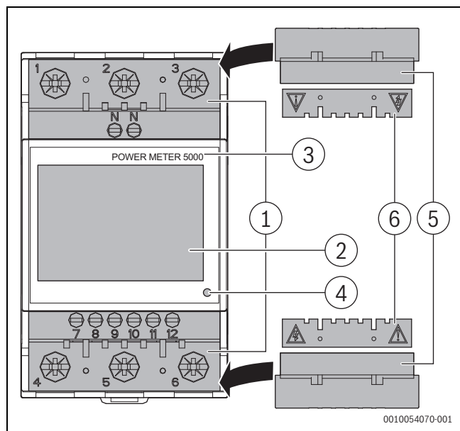
Fig. 382 Prezentare generală a produselor
