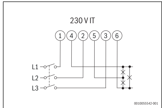
Fig. 235 Schema dell'impianto trifase, 3 fili conduttori (230 V IT)
