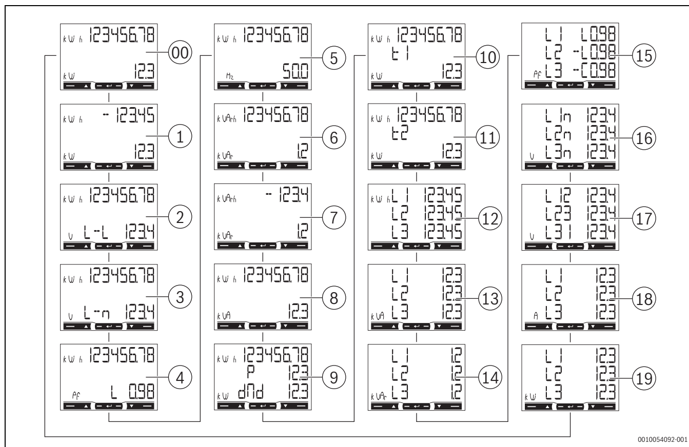
Fig. 340 Måleverdisider på visningsskjermen
