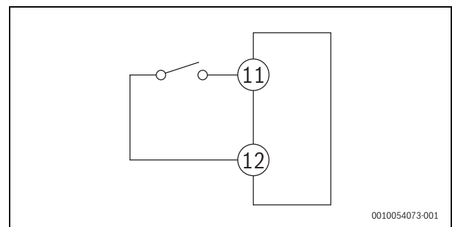
Fig. 122 Diagrama de entrada digital
