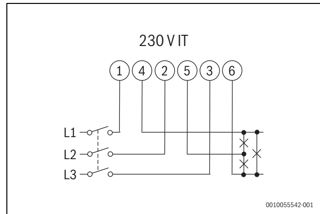
Bild 64 Anschlussplan Dreiphasensystem, 3 Leiter (230 V IT)
