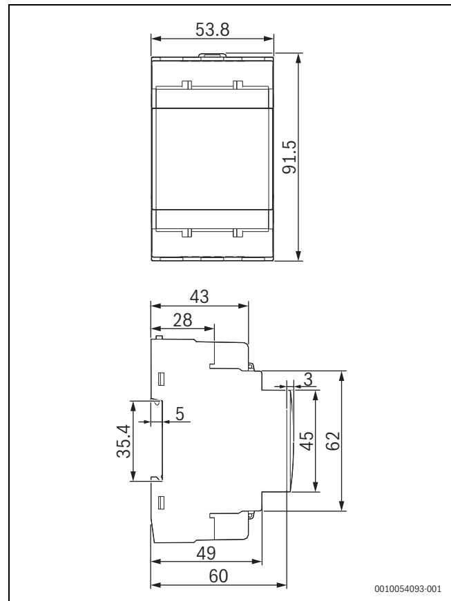
Afb. 289 Productafmetingen
