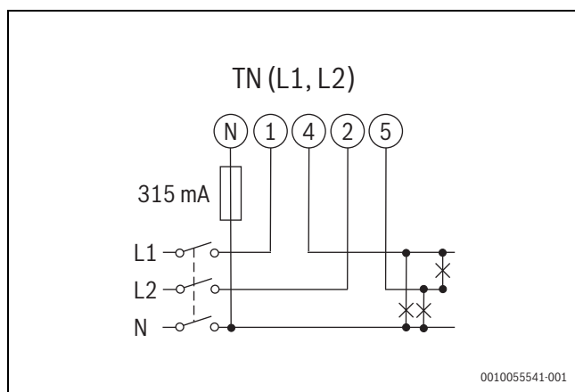
Fig. 177 Diagramme système biphasé, à 3 fils (TN)
