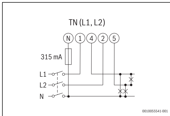
Kuva 158 Kaksivaiheinen järjestelmäkaavio, 3 johdinta (TN)
