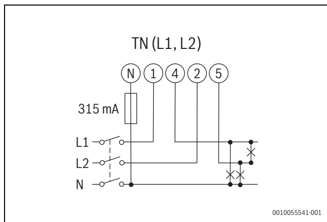
Bild 462 Diagram för tvåfassystem, 3-kablars (TN)
