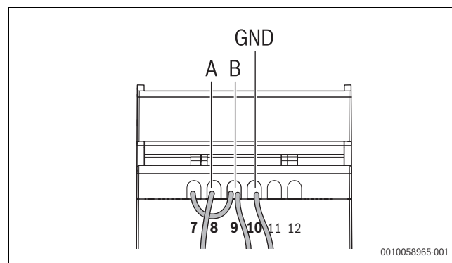
Sl.447 GND povezava
