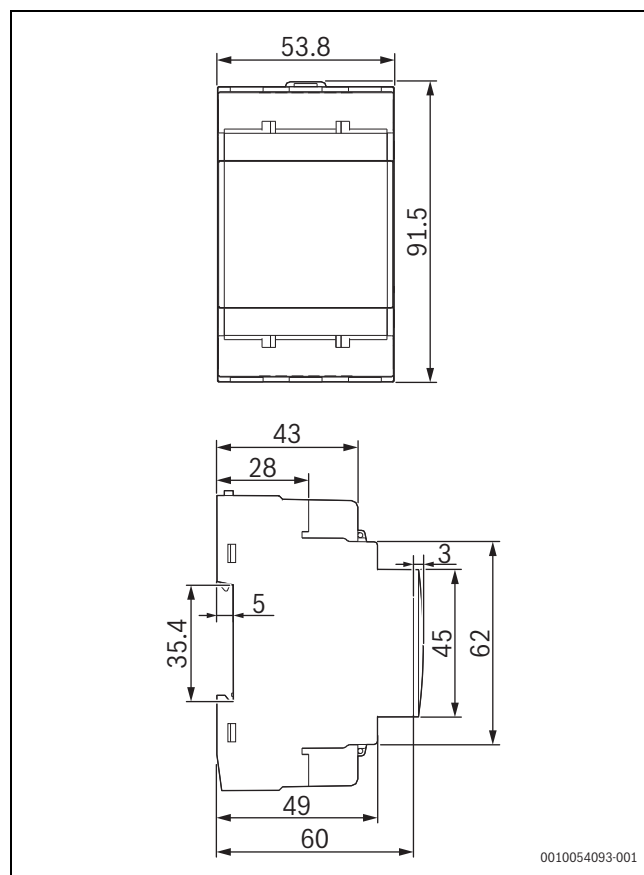
Pav. 270 Gaminio matmenys
