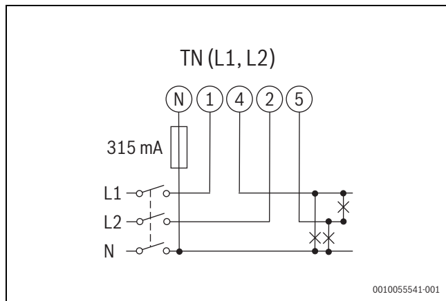
Σχ. 82 Διάγραμμα διφασικού συστήματος, 3 καλώδια (TN)
