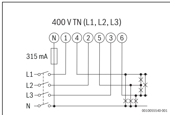
Joon. 138 Kolmefaasilise süsteemi graafik, 4 elektrijuhti (400 V TN)
