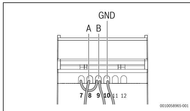
Фиг. 10 GND връзка
