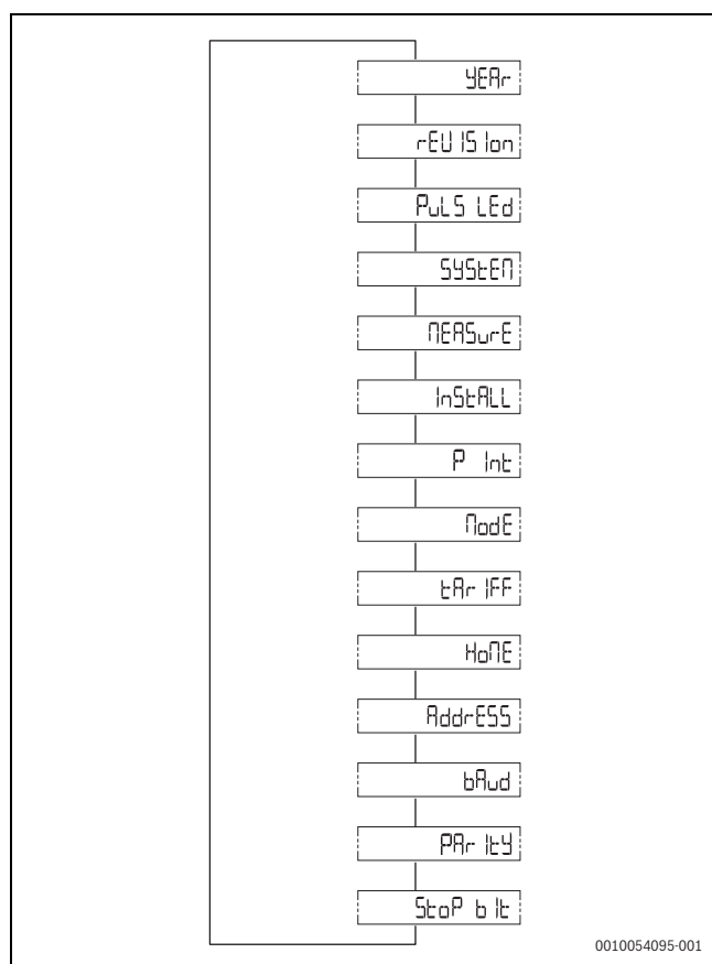
Fig. 342 Informasjonsmeny på visningsskjermen
