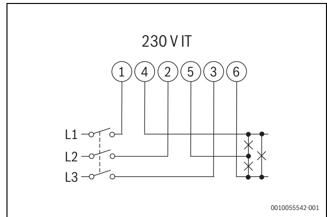
Fig. 121 Diagrama del sistema trifásico, 3 conductores (230 V IT)
