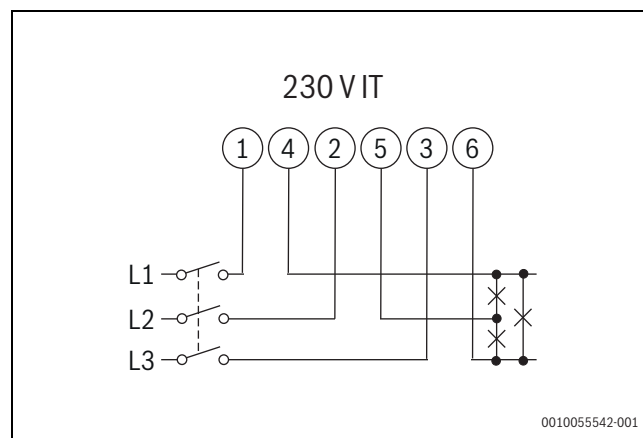
Fig. 387 Diagramă sistem trifazat, cu 3 fire (230 V, IT)
