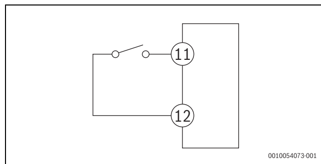
Obr. 27 Schéma digitálního vstupu
