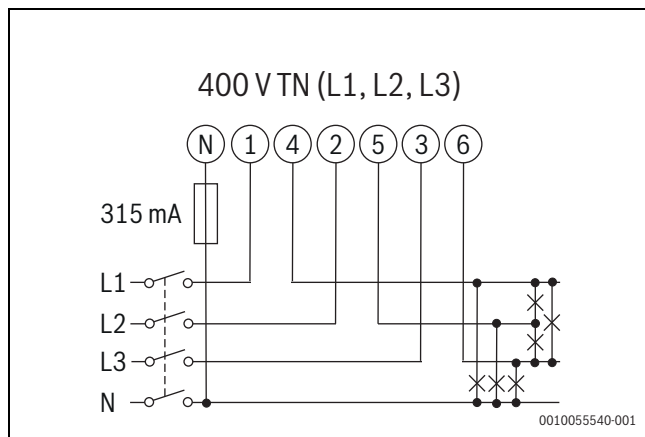
sl. 404 Trofazni sistem Dijagram, 4-žičani(400 V TN)
