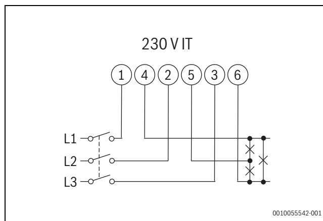
Fig. 368 Diagrama do sistema trifásico, 3 condutores (230 V IT)
