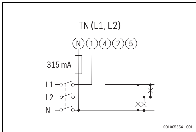
Мал. 481 Схема з'єднань двофазної системи, 3 жили (TN)
