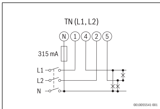
Rys. 348 Schemat systemu dwufazowego, 3-żyłowy (TN)
