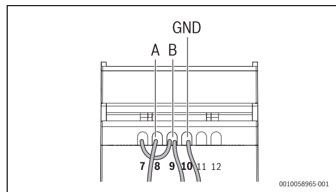
Fig. 48 GND-forbindelse
