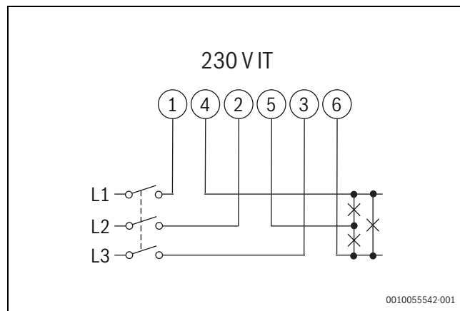
Afb. 292 Driefase systeem diagram, 3-draads (230 V IT)
