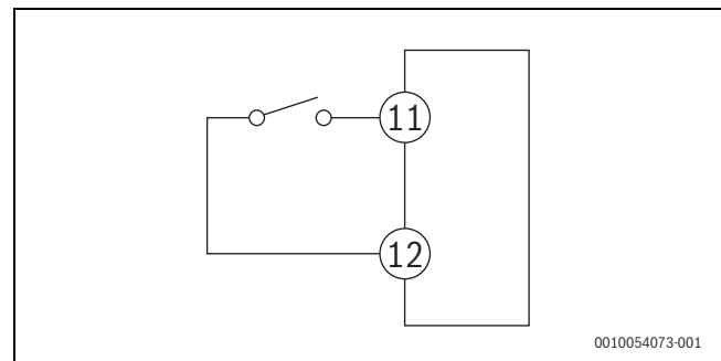
Kuva 160 Digitaalitulon kaavio
