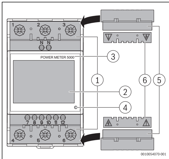
Kuva 154 Tuotteen yleiskuvaus
