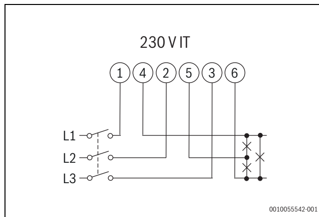
Fig. 178 Diagramme système triphasé, à 3 fils (230 V IT)
