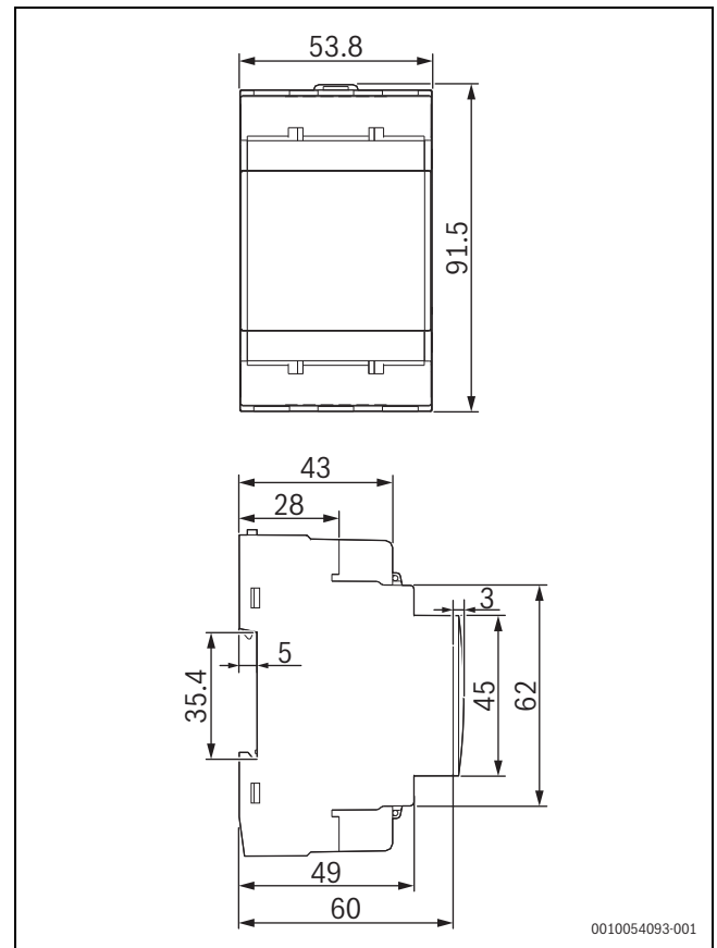
Σχ. 80 Διαστάσεις προϊόντος
