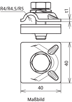
Maßbild
