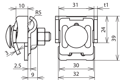
Maßbild FK KB 6.10 KBF0.7 8 CU
