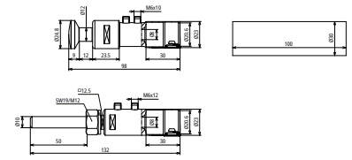
Maßbild HVI LO ASS RIV KF V2A
