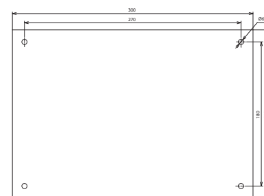
Maßbild HWS 300X210 AGBS HVI DE EN K
