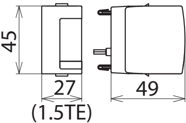
Maßbild DG MOD DC Y 500
