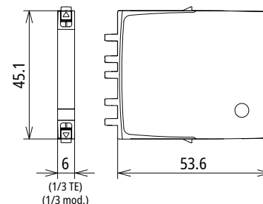
Maßbild BCO MOD ML2 BD 48
