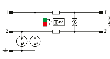
Prinzipschaltbild BCO MOD ML2 BD 48
