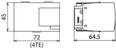
Maßbild DV MOD TNS 255
