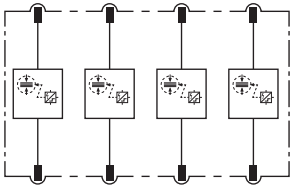
Prinzip Schaltbild DV MOD TNS 255
