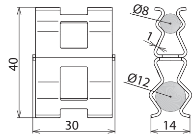
Maßbild DC BK 8 RD12 STBLANK
