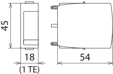
Maßbild DG MOD H A NPE
