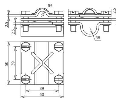
Maßbild KS 16 8.10 FL30 OV ZP CU
