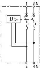
Prinzipialschaltbild POP 2 255 C25
