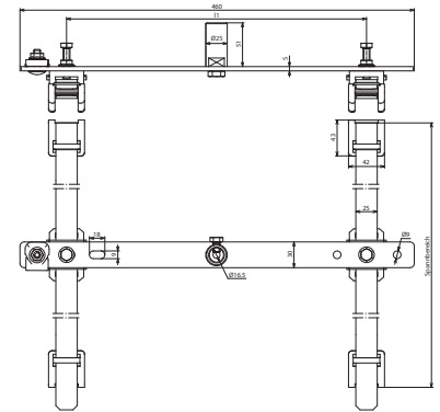
Maßbild HA 16 2F FG120.300 V2A
