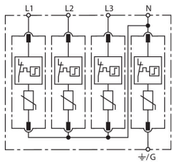
Prinzipschaltbild DG MU 3PY 600 4W+G
