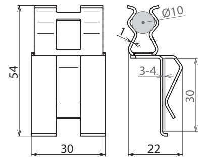
Maßbild DC BK 10 FL30 STBLANK
