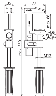
Maßbild ZK85 BS
