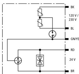
Prinzip Schaltbild DPI CD EXD 230 24 N
