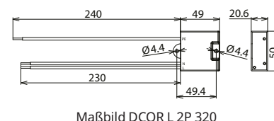
Maßbild DCOR L 2P 320
