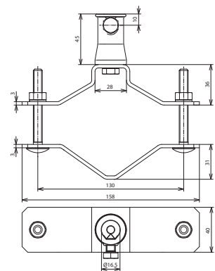
Maßbild RS D70.90 BB16 V2A ZG
