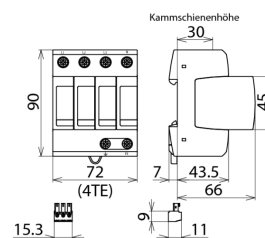
Maßbild DG M TT 385/305 FM
