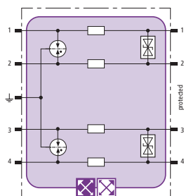
Prinzipschaltbild BXT ML4 BD HF 5
