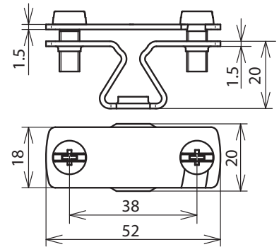
Maßbild FBH ZS 30 M8 V2A
