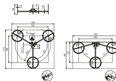
Maßbild DBS KB D40.50 RA560 STTZN
