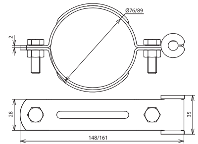
Maßbild LH KD 8.10 D76 STTZN
