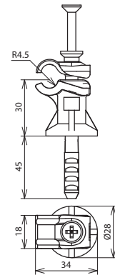
Maßbild LH DFI DQ 6.10 CU H30 BR
