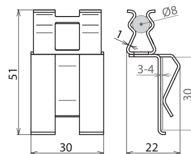
Maßbild DC BK 8 FL30 STBLANK
