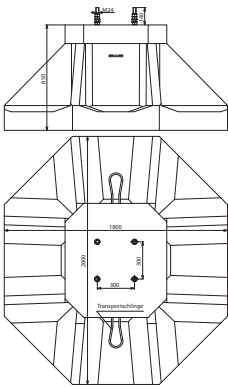
Maßbild KÖFU I TBM FP400
