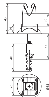
Maßbild LH DG 8 H20 HS5X50 KD8 CU BR
