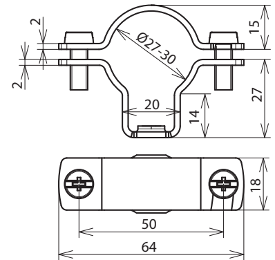
Maßbild LH ZS 27 GM6 V2A
