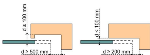
Ábra 2: Biztonsági távolság
