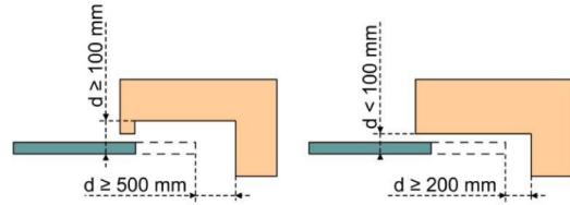
Şekil 2: Güvenlik mesafesi
