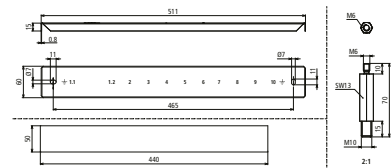
Maßbild PAS EX AD 11 AP
