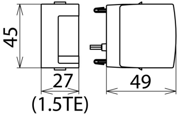
Maßbild DG MOD E DC 900
