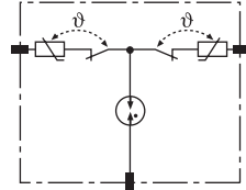
Prinzipschaltbild DR MOD 60
