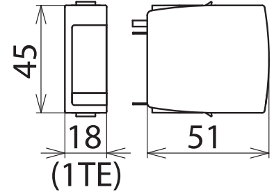
Maßbild DR MOD 60
