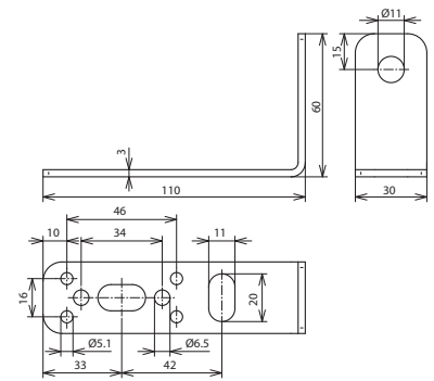
Maßbild BW90 B11 B5.1 6.5 11 V2A
