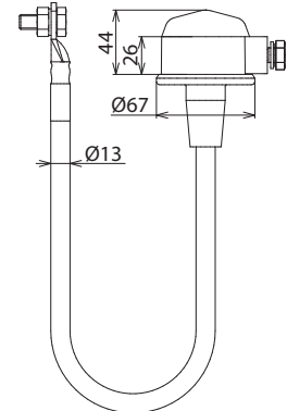
Maßbild EXFS L200
