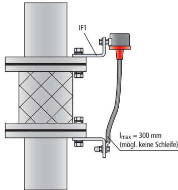
Prinzipschaltbild EXFS L200
