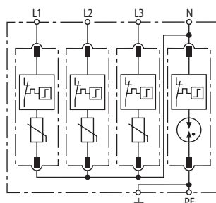
Prinzipialschaltbild DG M TT 385
