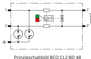
Prinzipschaltbild BCO CL2 BD 48
