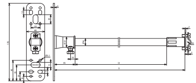
Maßbild DIDH 7.10 1030 BP V2A GFK
