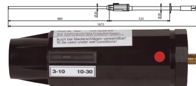
Maßbild PHE3 U 3 30 S
