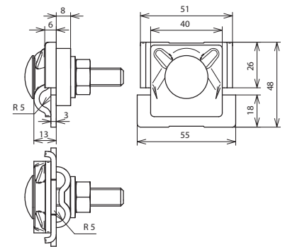
Maßbild FSK 3X8.10 FRM10X50 AL
